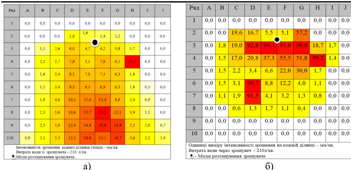
Рис. 2. Розподіл води: а) на горизонтальній площі зі зрошувача за горизонтальної його орієнтації у просторі, б) на горизонтальній площі зі зрошувача за вертикальної його орієнтації у просторі.
