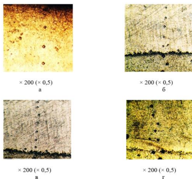
Рис. 1. Вплив ДФДЗ на структуру вуглецевих сталей з різним вмістом вуглецю після попереднього гартування. Режим ДФДЗ: S = 30 мм/с; t = 0,7 мм: а – сталь 20; б – сталь 45; в – сталь У7; г – сталь У12.
