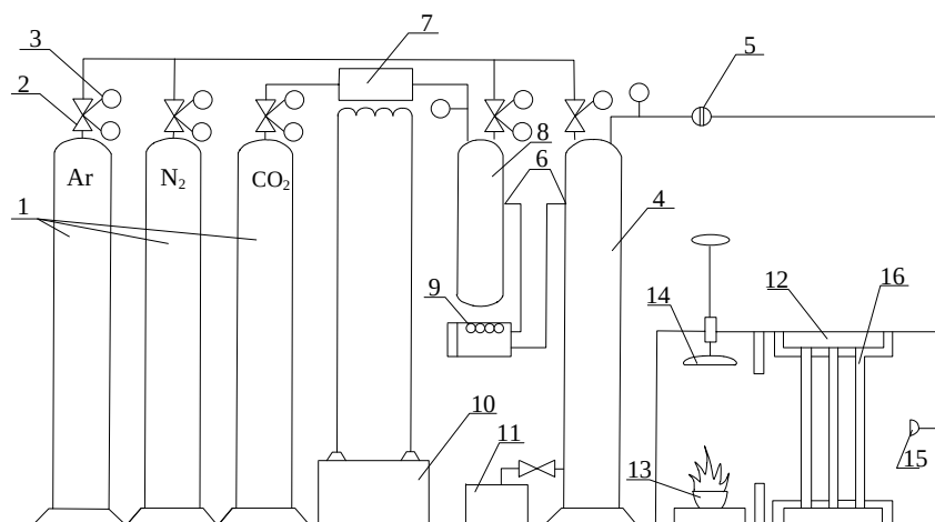
Рис. 1. Принципова схема лабораторного випробувального стенду: 1 – балон з газом; 2 – вентиль; 3 – манометр; 4 – змішувач; 5 – пробковий вентиль; 6 – термопари; 7 – випаровувач; 8 – накопичувач; 9 – регулювальний прилад; 10 – трансформатор; 11 – блок продувки; 12 – випробувальна камера; 13 – модельне вогнище; 14 – пристрій гасіння; 15 – завихрювач; 16 – зразки.
