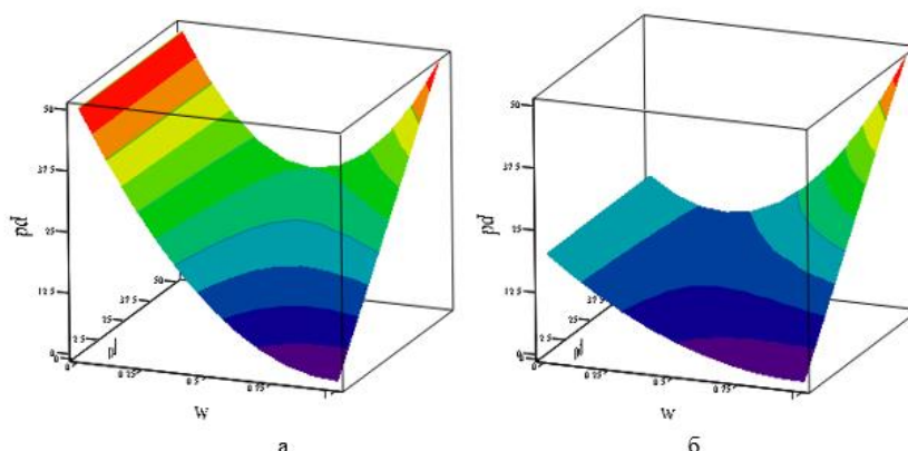
Рис. 1. Поверхні відгуку дисперсійної складової ВПЕ полімерних композитів \gamma_s^d від \omega та \gamma_p^d наповнювачів для полімерів з а – \gamma_f^d=50 мДж/м 2 ; б – \gamma_f^d=20 мДж/м 2 .
