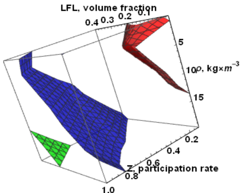
Рис. 1. Зображення, отримані за допомогою функції FE. Межа розділу простору з небезпечними та безпечними об'єктами: \rho – густина газу, \text{kg}\cdot\text{m}^{-3} ; LFL – нижня концентраційна межа поширення полум'я, об'ємна частка; Z - коефіцієнт участі газу в горінні; LFL – нижня межа поширення полум'я в об'ємних частинах. Червона поверхня відповідає значенню критерію небезпеки -10. Синя поверхня відповідає значенню критерію небезпеки 0. Зелена поверхня відповідає значенню критерію небезпеки 170.
