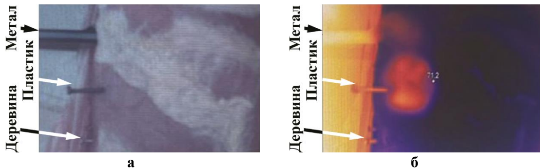
Рис. 2. Результати обробки отриманих під час вимірювань з використанням методів кореляційної НВЧ гіпертермії та проєкційної динамічної теплової томографії даних: а – у видимому діапазоні; б – в ІЧ-діапазоні.
