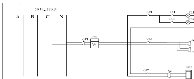
Рис. 1. Схема типової квартирної електромережі.
