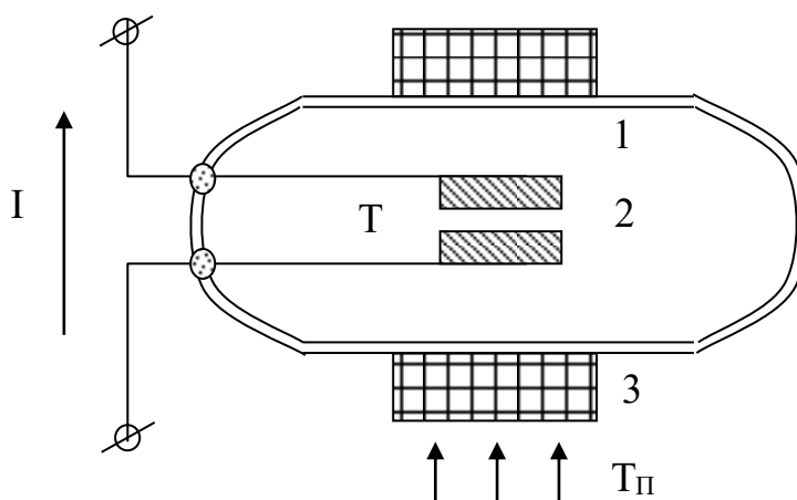
Рис. 1. Розрахункова схема магнітноконтатного чутливого елемента: 1 – геркон; 2 – контакти; 3 – кільцевий постійний магніт.
