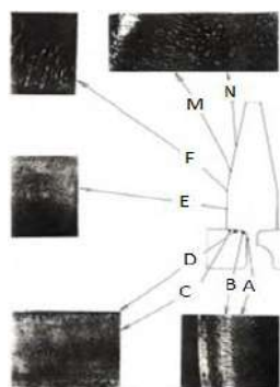
Рис. 2. Пошкодження піки та втулки, зміцнених детонаційним напиленням, \times 3 .
