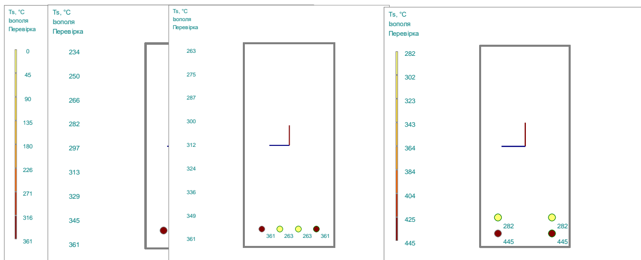
Рис. 1. Температура в арматурі для різних схем армування перерізу балки.
